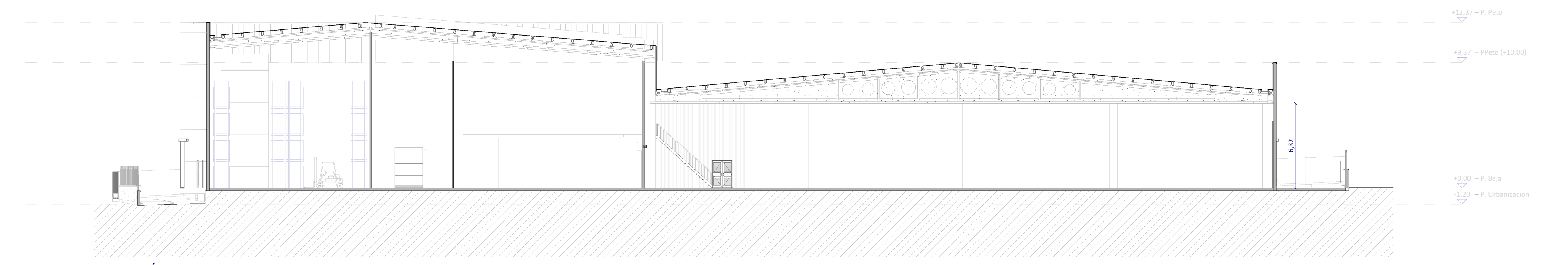
C- SECCIÓN 1:200
