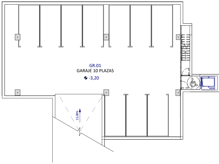
PLANTA SEMISÓTANO 1 : 200
