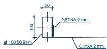
PLANTA DETALLE A Escala 1/10
