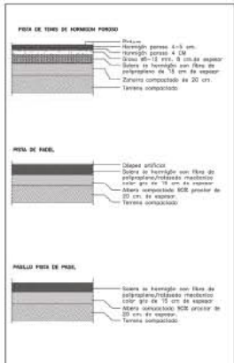
DETALLES CONSTRUCTIVOS. ESCALA 1/20
